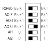
Рисунок 8.5 – Положение переключателей
